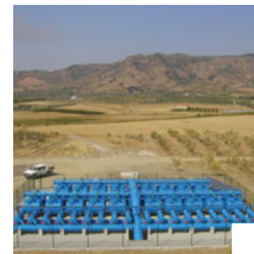
Réseaux d'irrigation et de drainage, système de pompage et d'amenée de l'aménagement hydro-agricole de Vale da Vilarica
