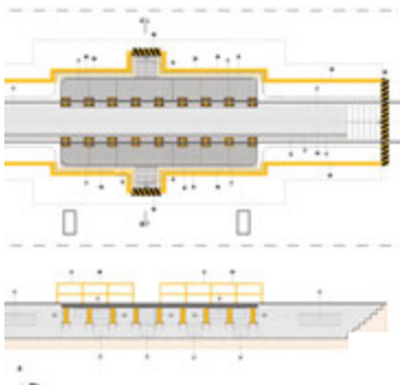
Digue pour la maintenance du matériel roulant. Cascais, Portugal EMEF - Empresa de Manutenção de Equipamento Ferroviário, SA Projet, inclus Avant Projet Sommaire, Avant Projet Détaillé, DAO et Assistance technique maîtrise d'ouvrage.
